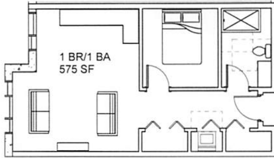
3 1 BR TYP SCALE: 1/8" = 1'-0"
