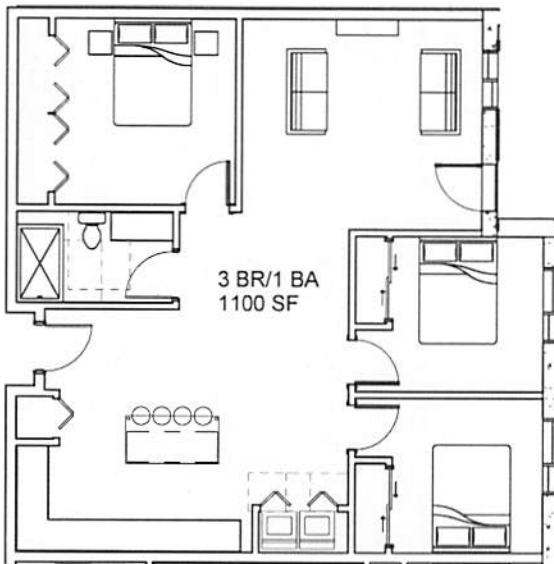
2 3 BR, TYP SCALE: 1/8" = 1'-0"
