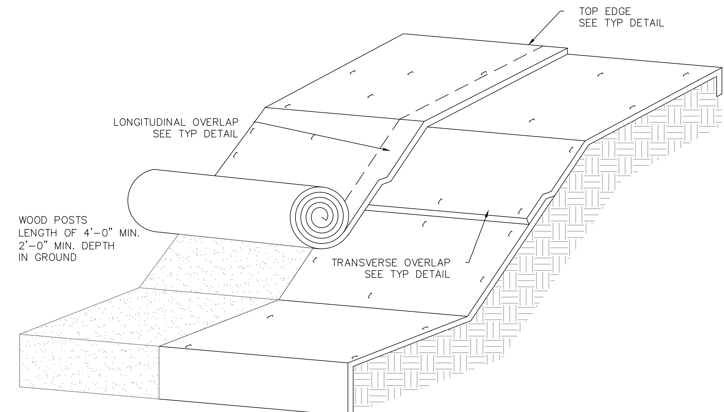
TOP EDGE TYP DETAIL
