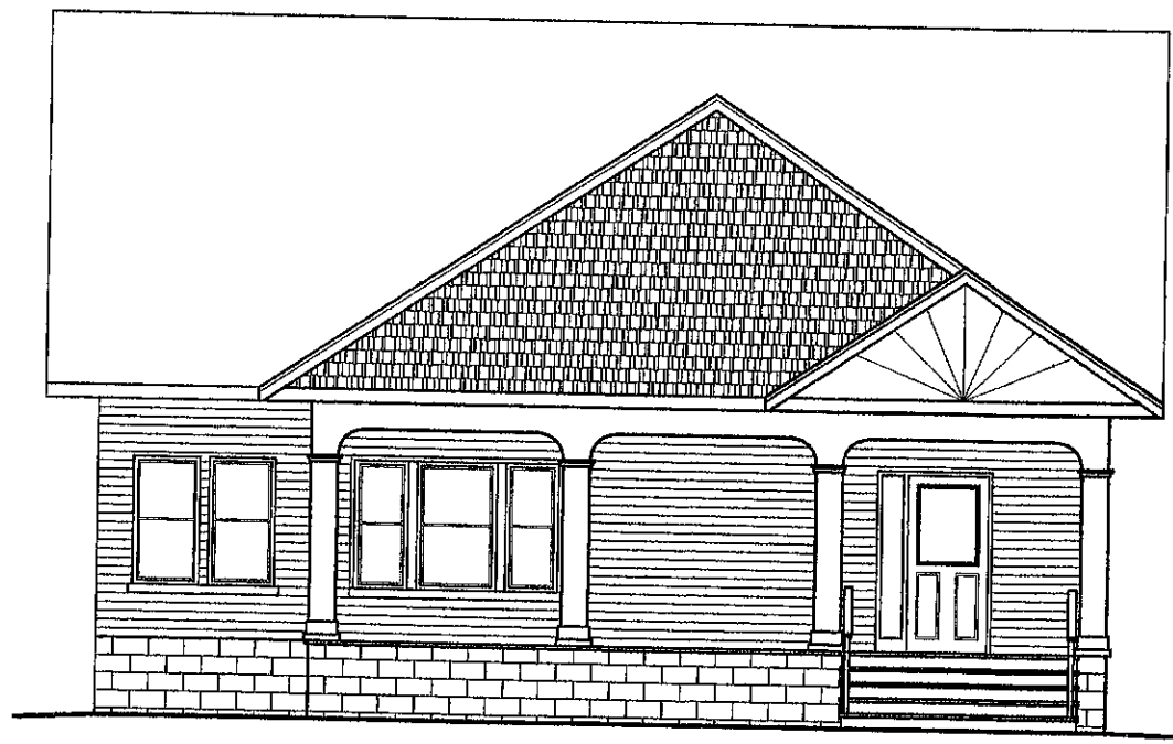
2 A2 EXTERIOR ELEVATION 1/8" = 1'-0"
