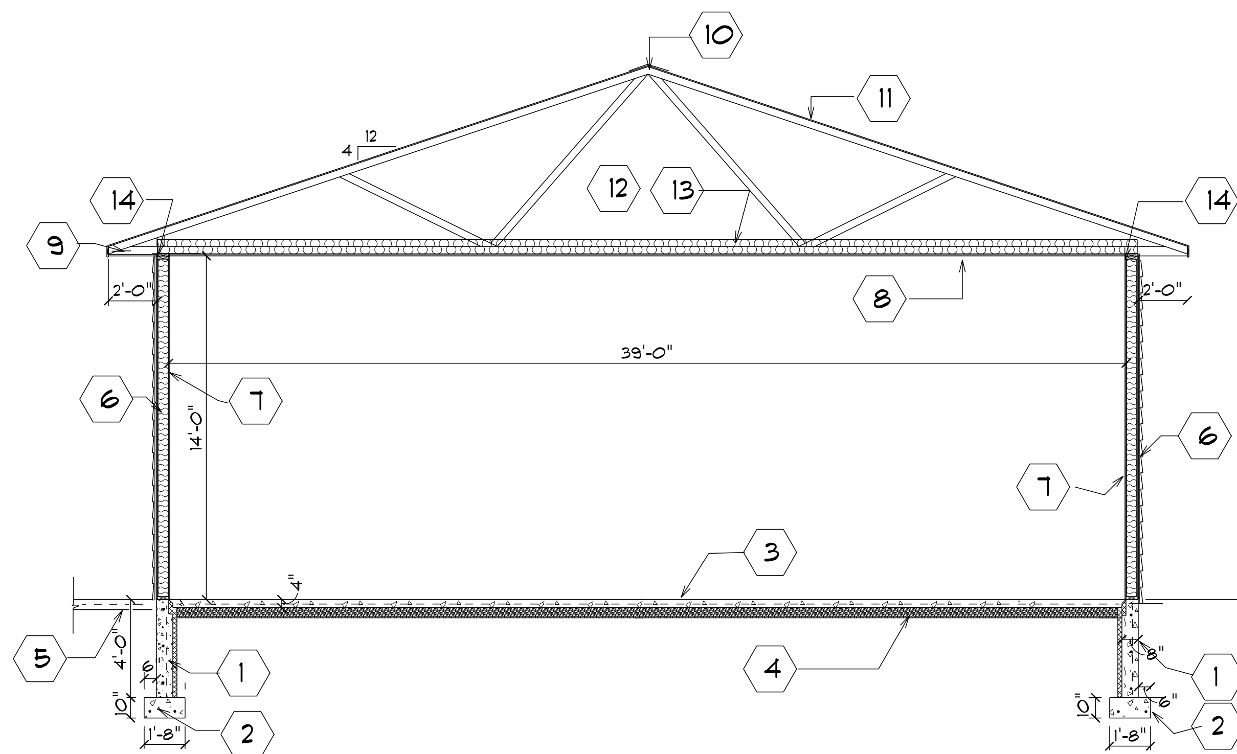
AA A4 SECTION 1/4" = 1' - 0"
